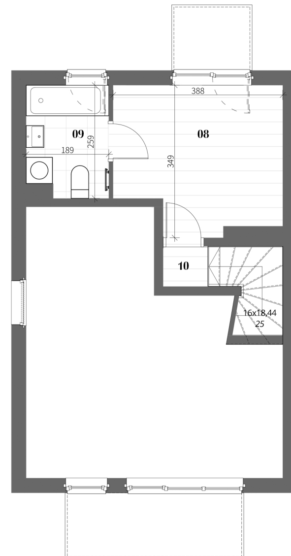
1. PIĘTRO
